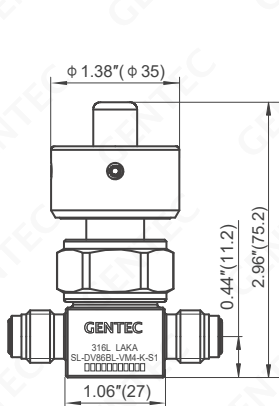
Handgrip (300 psi)
