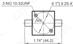
TW6
