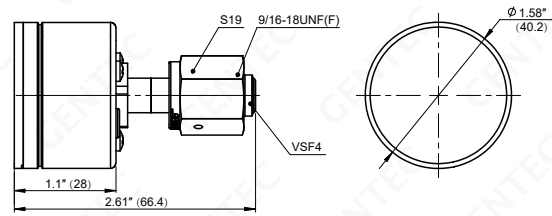
GUR15SL-*-VSF4
