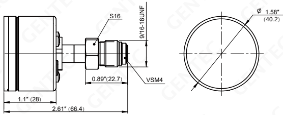
GUR15SL-*-VSM4
